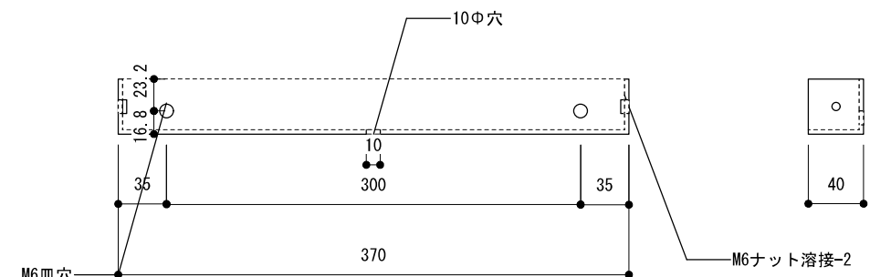
3 モニター側金物下部 縮尺: 1:5
